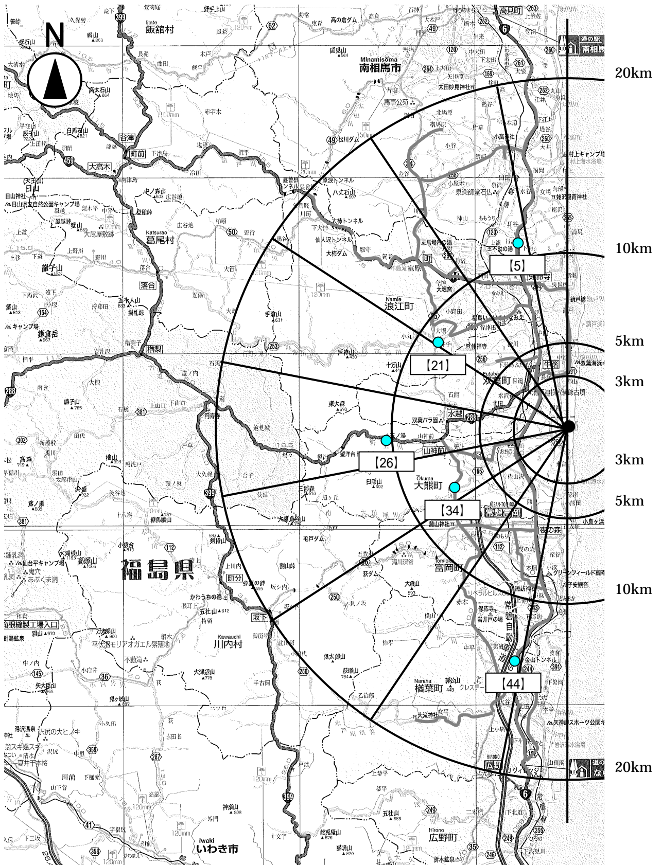
東京電力株式会社福島第一原子力発電所より20km圏内の空気中放射性物質濃度の試料採取ポイント（採取日：平成24年8月27日、28日）
